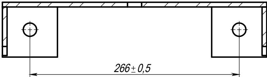
A-A (1 : 3)
